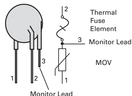
iTMOV® Varistor
