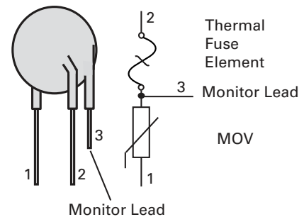
iTMOV® Varistor
