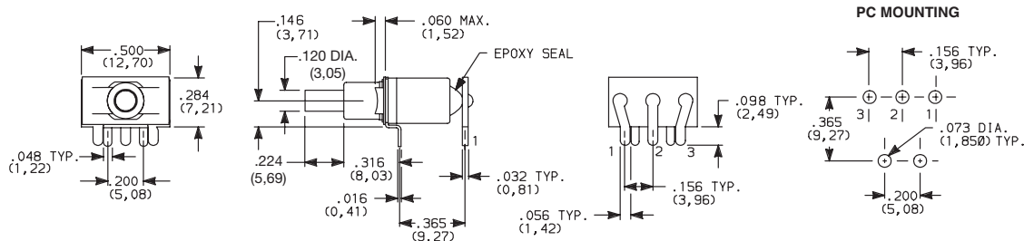
E112SD1R2BE SPDT
