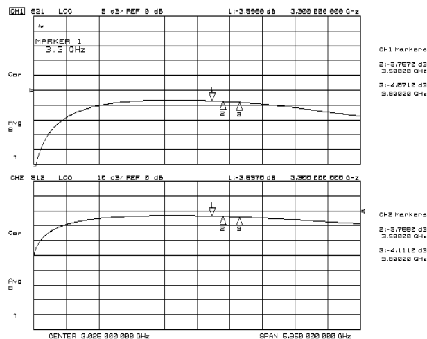
S21, S12
