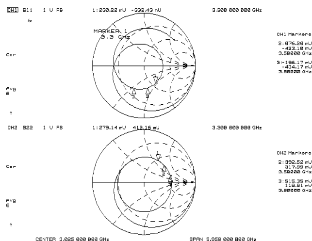
Zin, Zout
