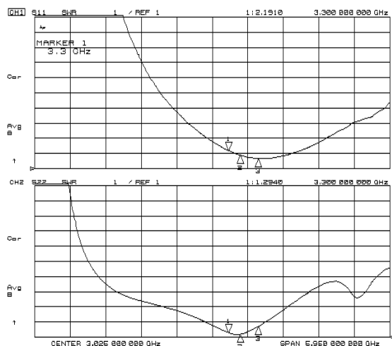
VSWRi, VSWRo
