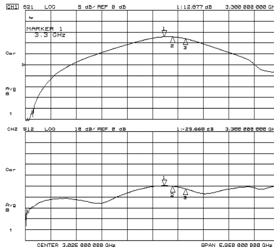
S21, S12
