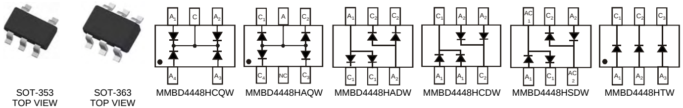
SOT353/SOT363
