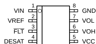
NCD5703C
