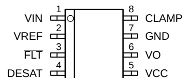
NCD5703A
