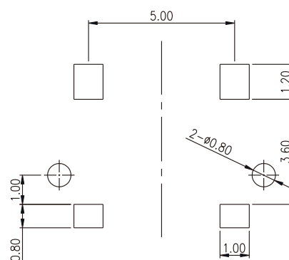
P.C.B. LAYOUT
