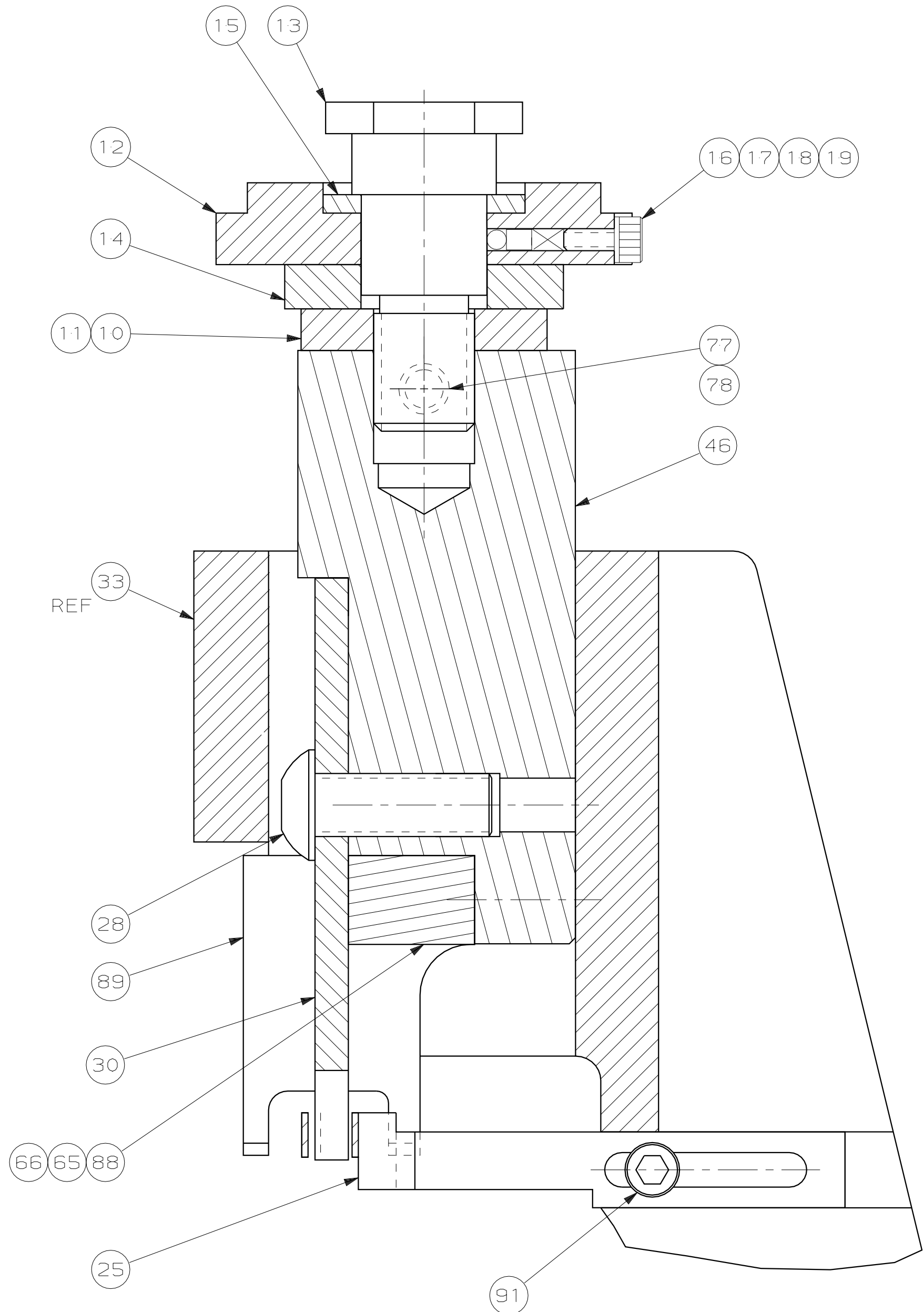
SECTION D-D
