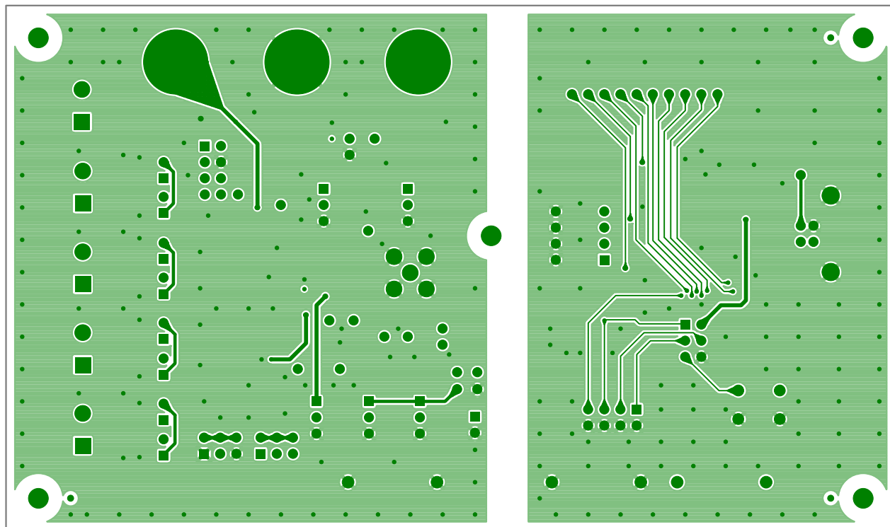
FIGURE 23. BOTTOM LAYER
