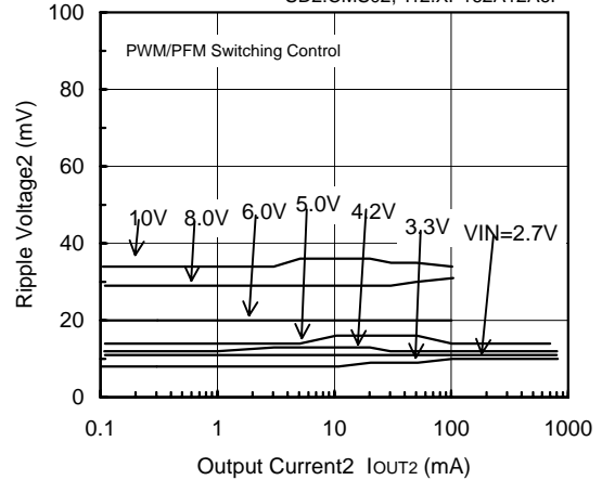
FOSC=300kHz, VOUT2=2.5V
