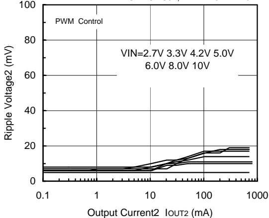
FOSC=300kHz, VOUT2=2.5V
