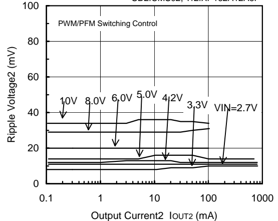
FOSC=300kHz, VOUT2=2.5V
