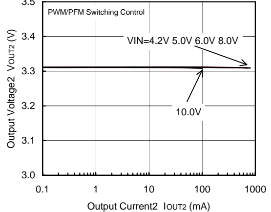
FOSC=300kHz, VOUT2=3.3V
