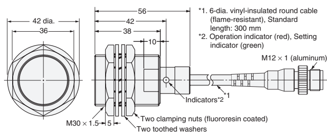
E2EQ-X10D1-M1(T)GJ
