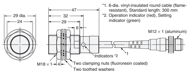
E2EQ-X7D1-M1(T)GJ
