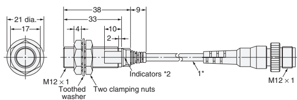
E2EQ-X4X1-M1(T)J
