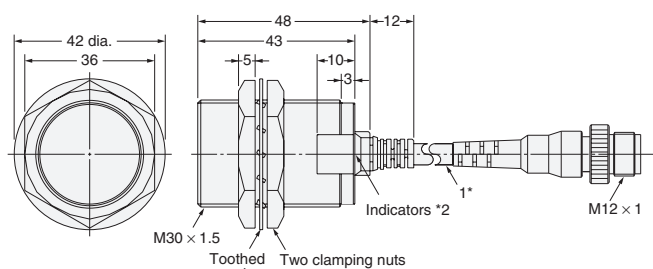
E2EQ-X15X1-M1(T)J
