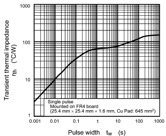
Fig. 7.12 r_{th} - t_w
