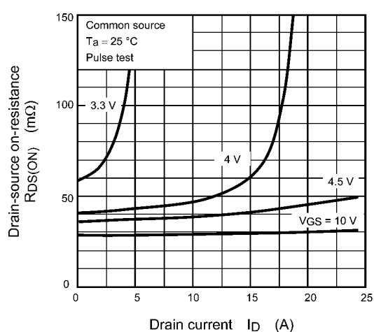
Fig. 7.4 RDS(ON) - ID
