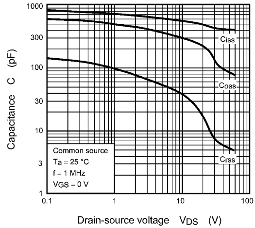
Fig. 7.8 C - V_{DS}
