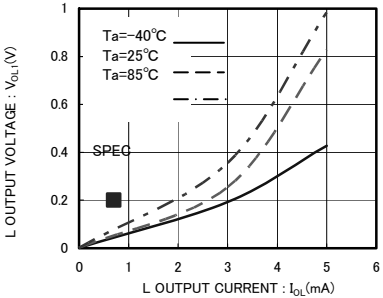
Fig.5 'L' output voltage V_{OL1-IOL} ( V_{CC}=1.7\text{V} )
