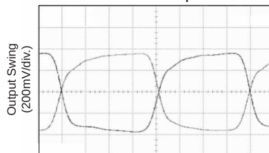
1.25GHz Output
