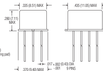
MGAT ENCLOSURE
