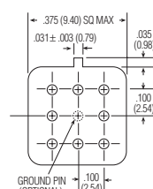
MGA/MGAD/MGADD HEADER
