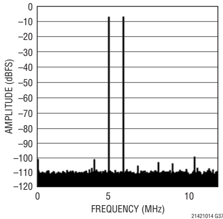
LTC2140-14: 64k Point 2-Tone FFT, f_{IN} = 69\text{MHz} , 70\text{MHz} , -7\text{dBFS} , 25\text{Mpsps}
