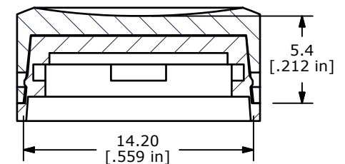
SECTION A-A SCALE 3:1
