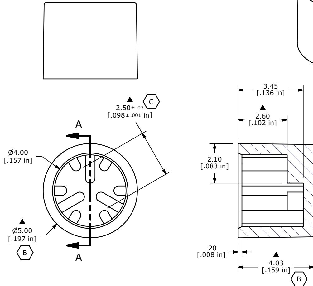
SECTION A-A SCALE 8 : 1
