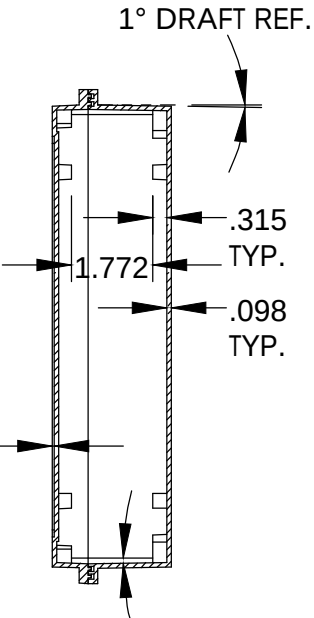
SECTION A-A
