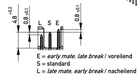
Stecklänge / mating length
