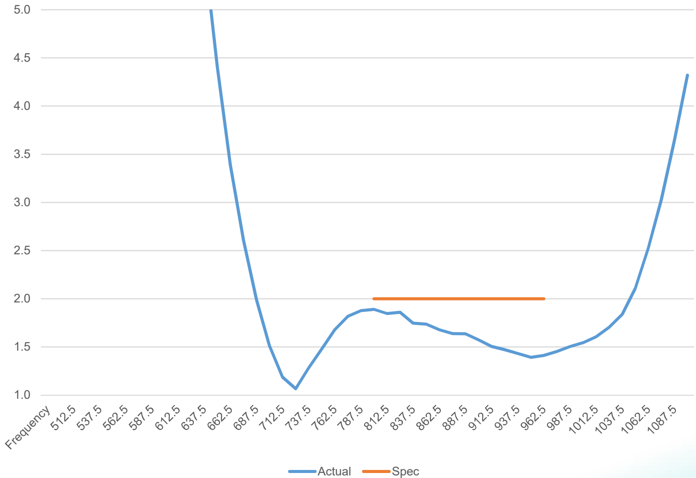
ICEFIN806NMO VSWR
