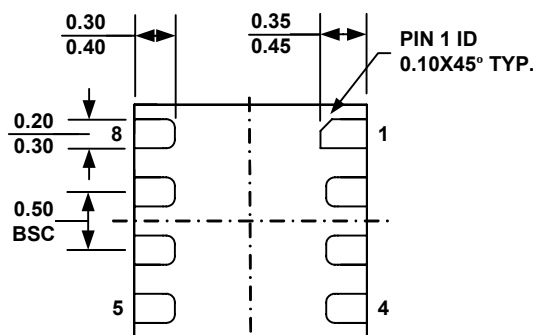
QFN8 (2mmx2mm)
