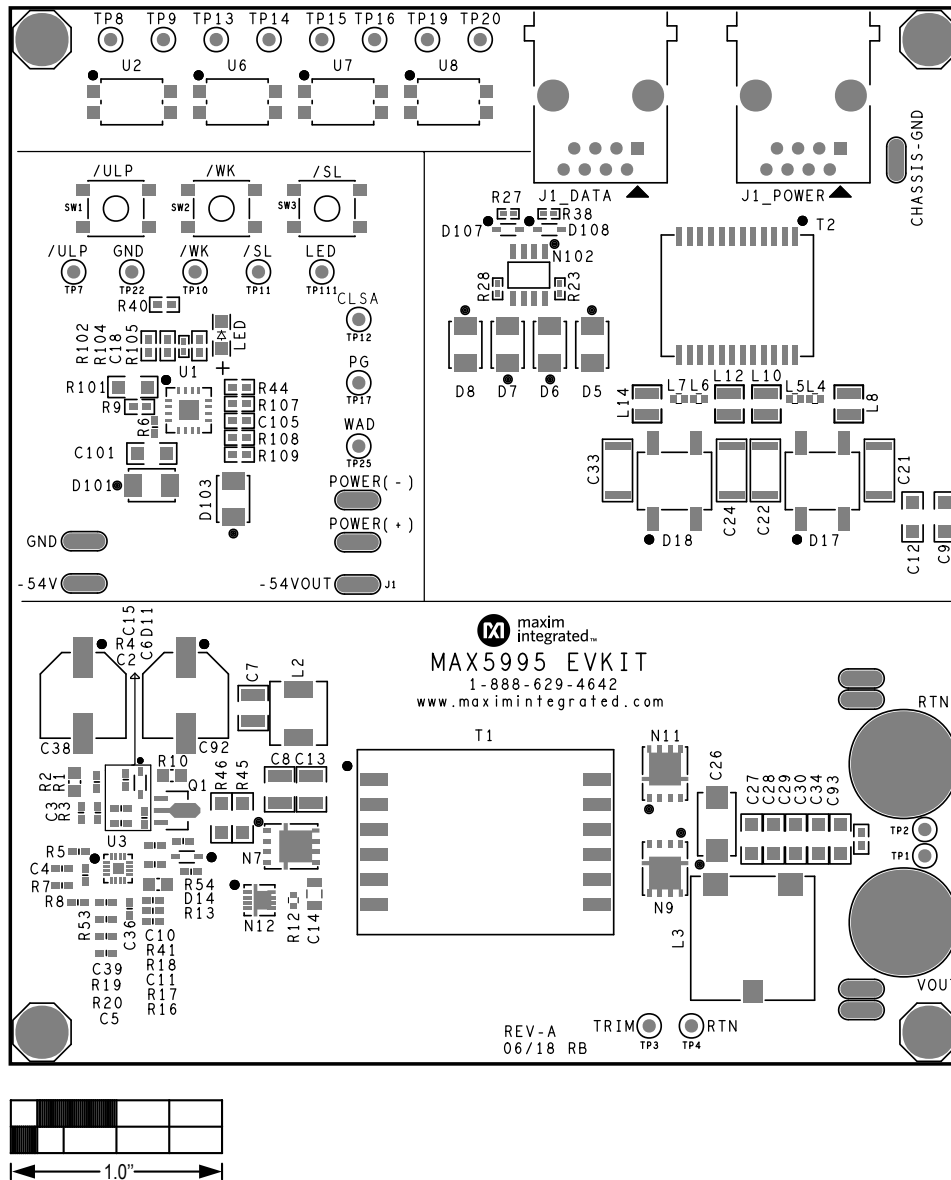
MAX5995 EV—Top Silkscreen
