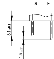
Stecklänge / mating length
