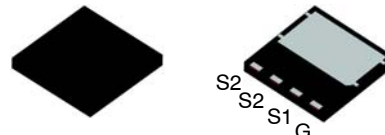
Power 88 PQFN4 8X8 2P CASE 483AP
