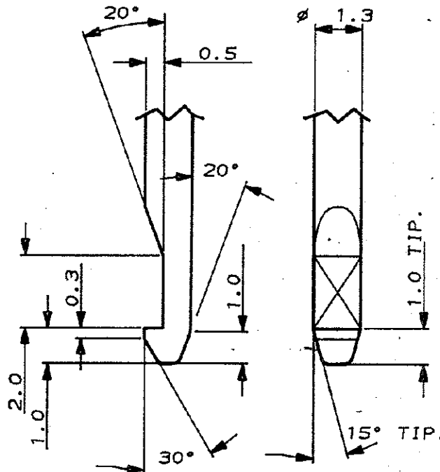
DETTAGLIO A
