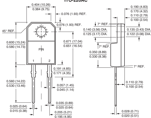
ITO-220AC
