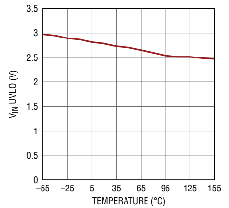
VIN UVLO
