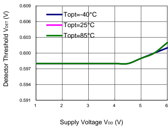
R3118x06xA/C
