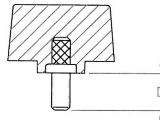
THREADED STUD
