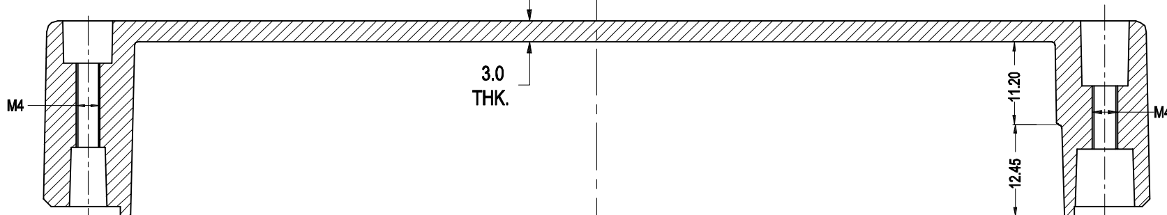
SECTION D-D
