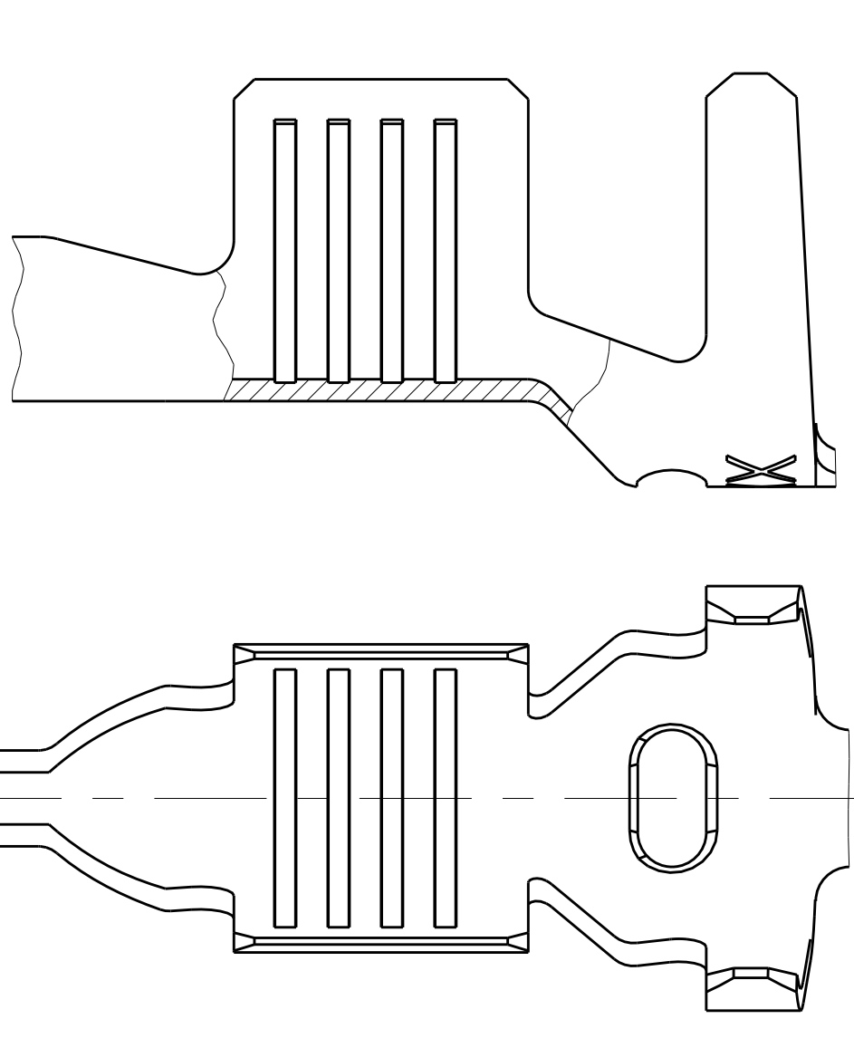
DESIGN 6 Ausfuehrung 6
