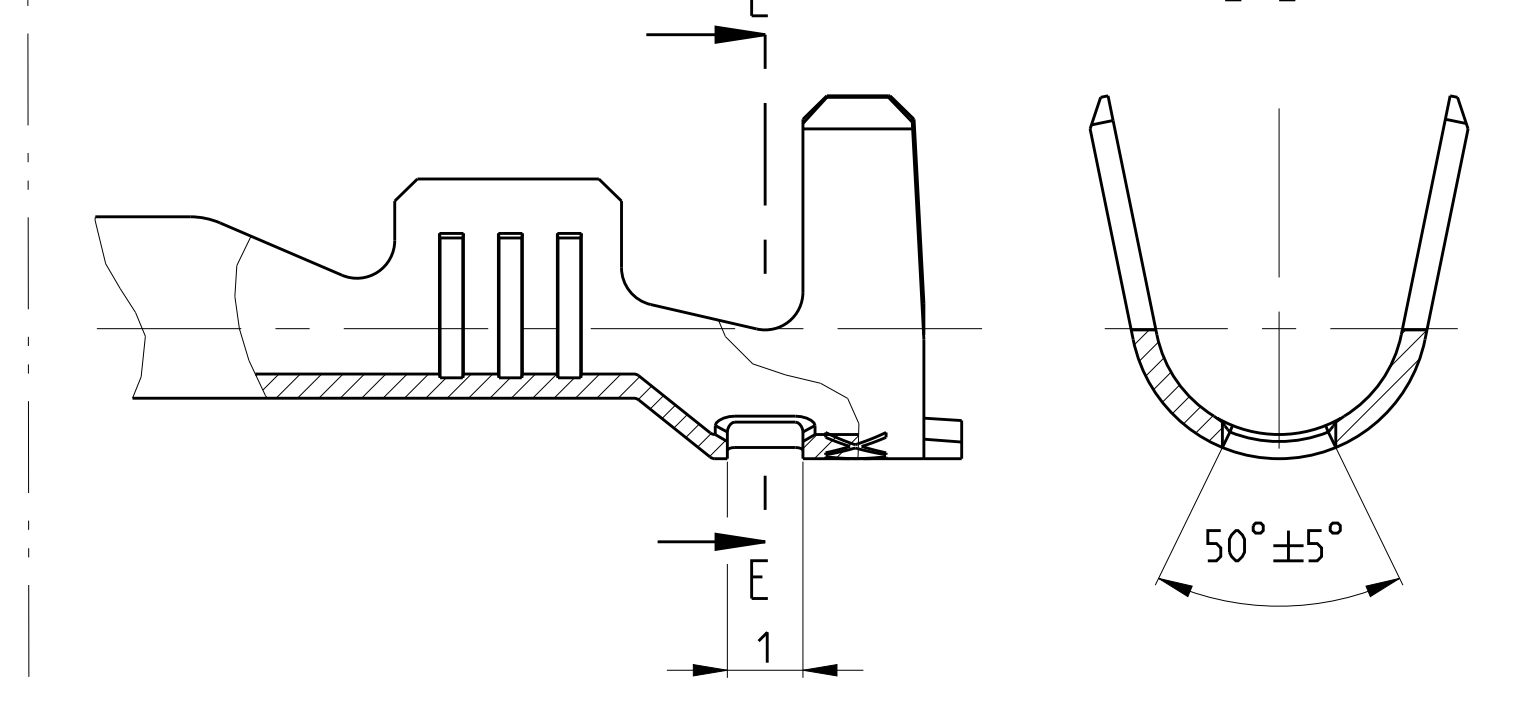
DESIGN 4 Ausfuehrung 4
