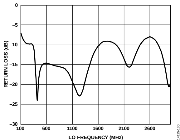
Figure 30. LO Return Loss
