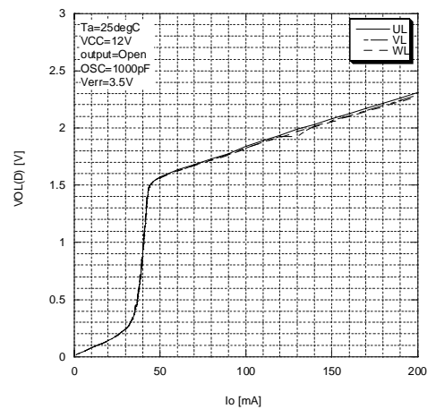
VOL(D) vs. Io
