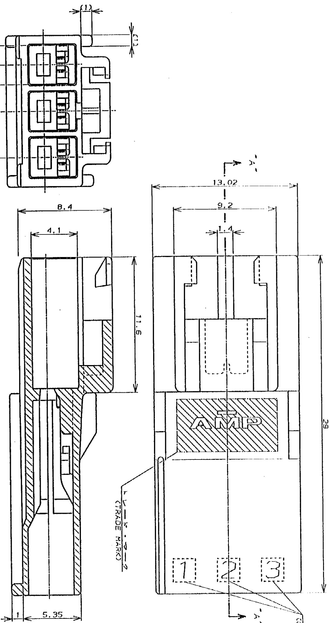
断面 A-A-A (SECT)
