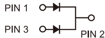
I²PAK
