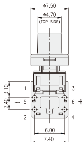
P.C.B. LAYOUT
