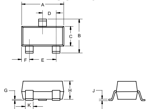
DIMENSIONS
