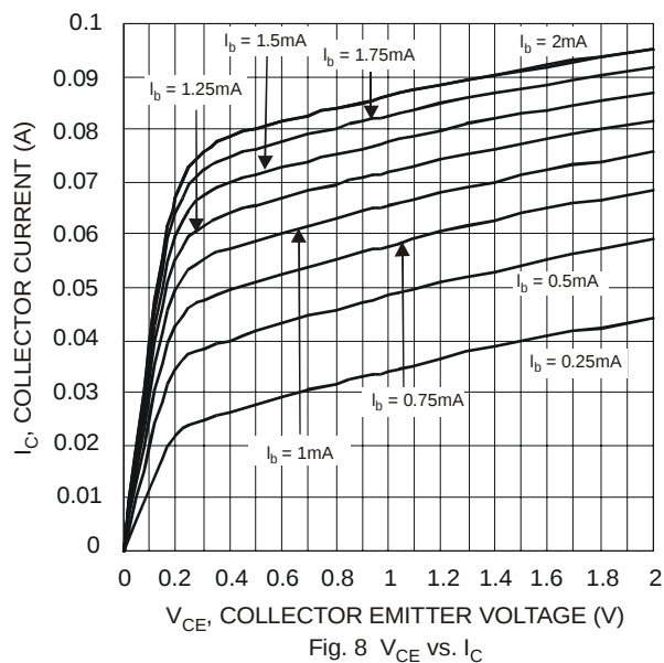
Fig. 8 V_{CE} vs. I_C
