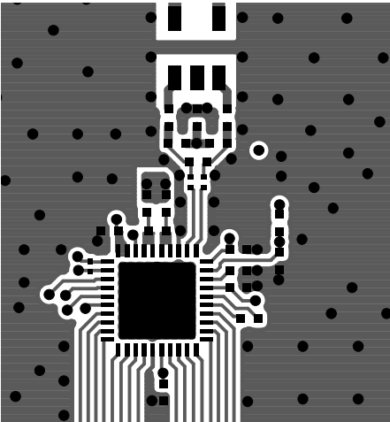
Top Side
