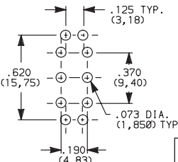
7201J1_BE2 DPDT
