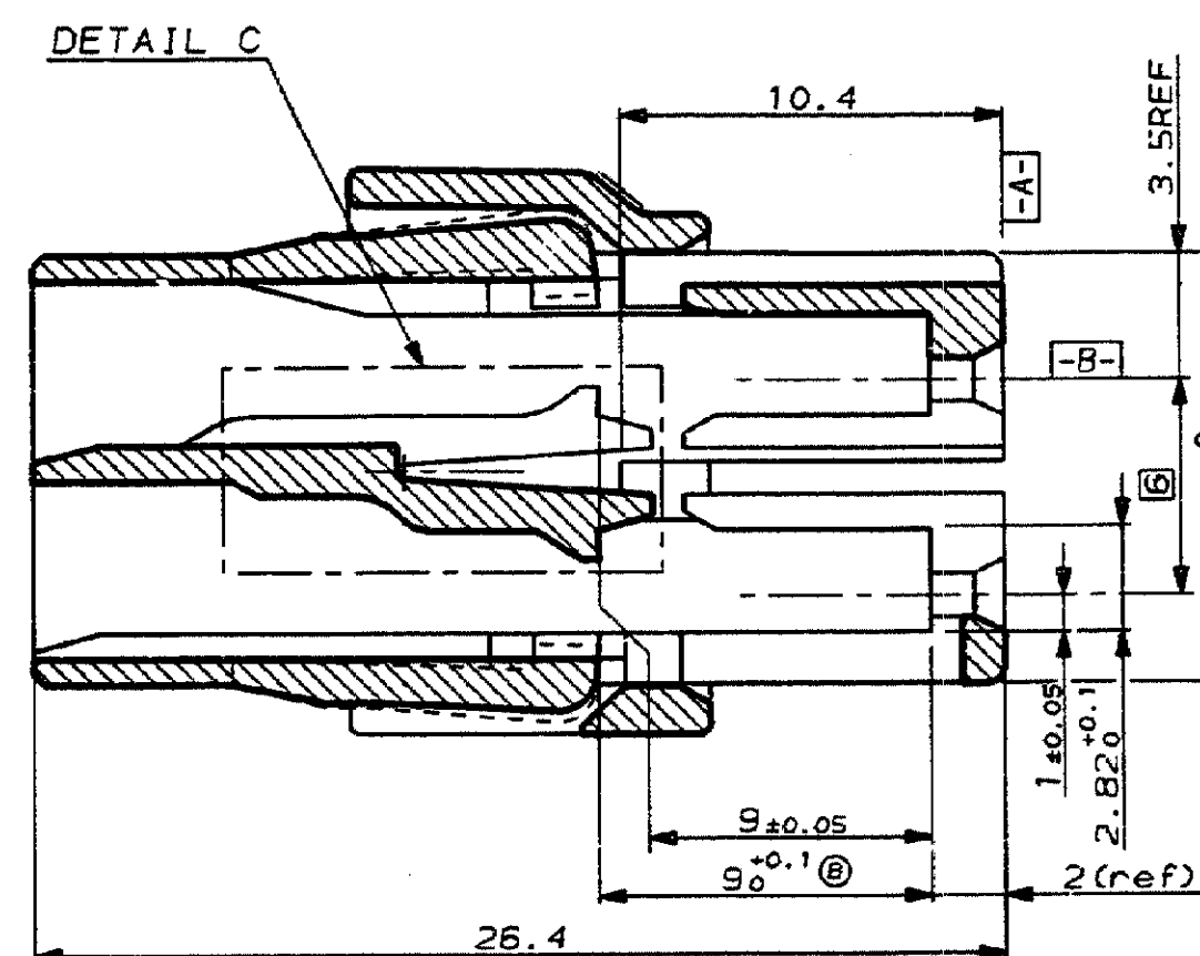
-COUPE BB-
