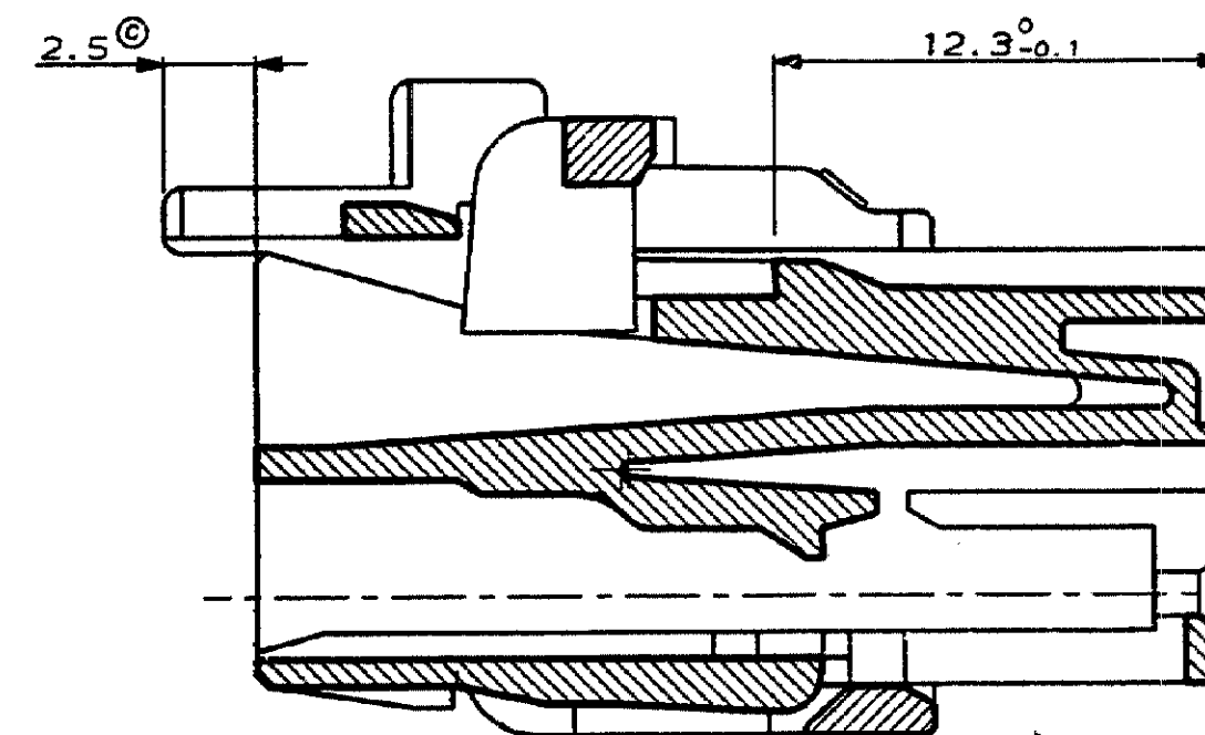
-COUPE AA-
