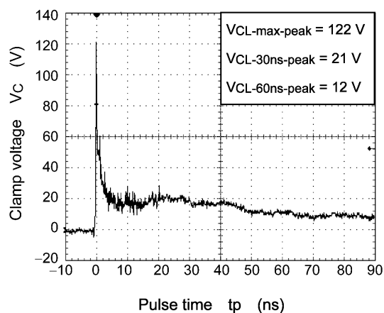
Fig. 6.1.1 +8 kV
