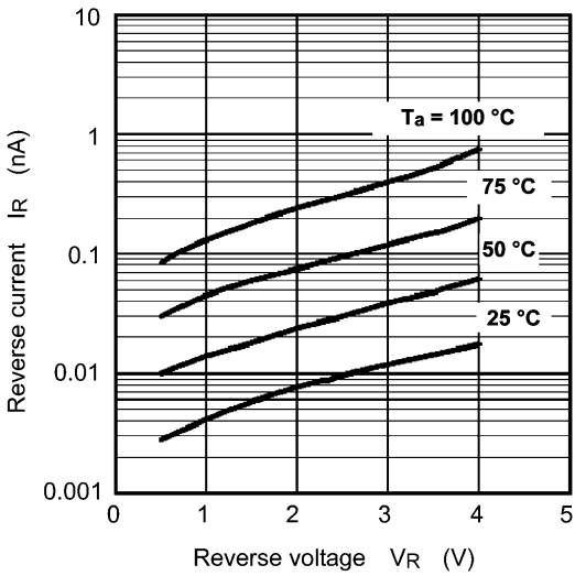
Fig. 9.2 I_R - V_R
