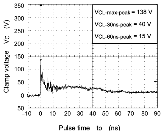
Fig. 6.1.3 +15 kV
