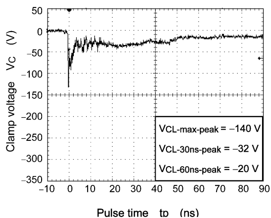
Fig. 6.1.4 -15 kV
