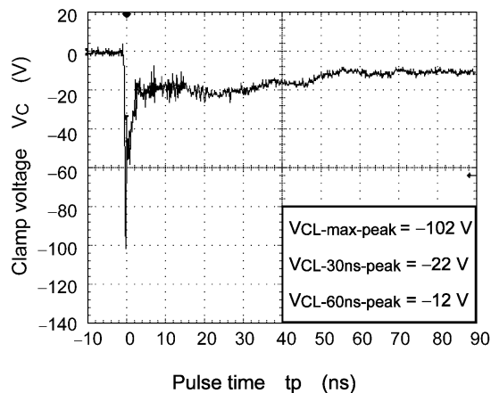
Fig. 6.1.2 -8 kV
