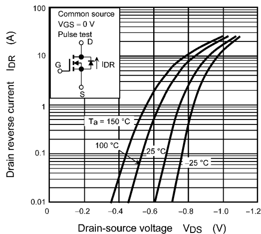
Fig. 8.7 I_{DR} - V_{DS}
