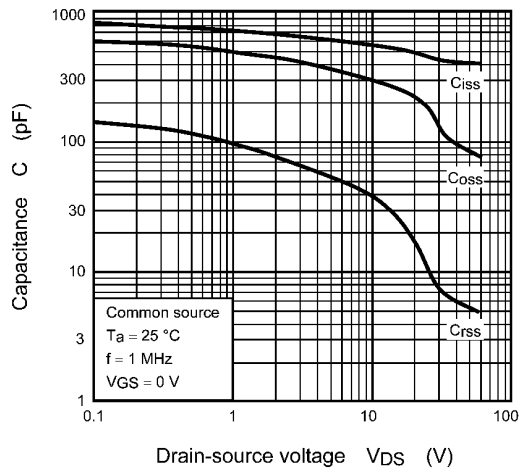
Fig. 8.8 C - V_{DS}
