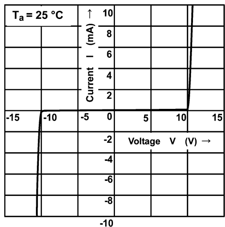
Fig. 9.1 I - V
