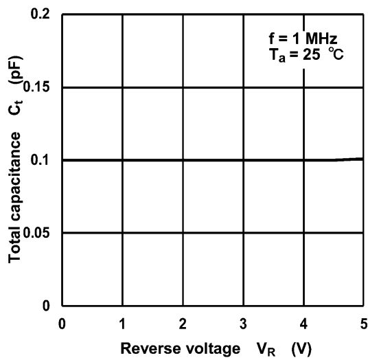
Fig. 9.3 C_t - V_R
