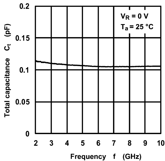
Fig. 9.4 C_t - f
