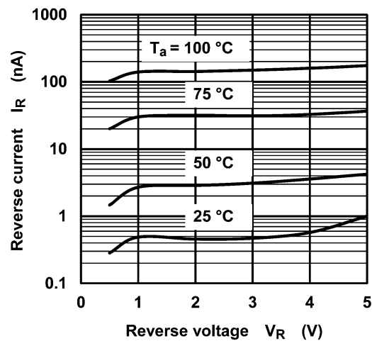
Fig. 9.2 I_R - V_R
