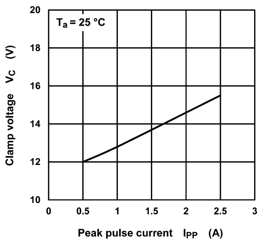
Fig. 6.2.1 V_C - I_{PP}
