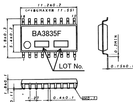
SOP18 (Unit:mm)
