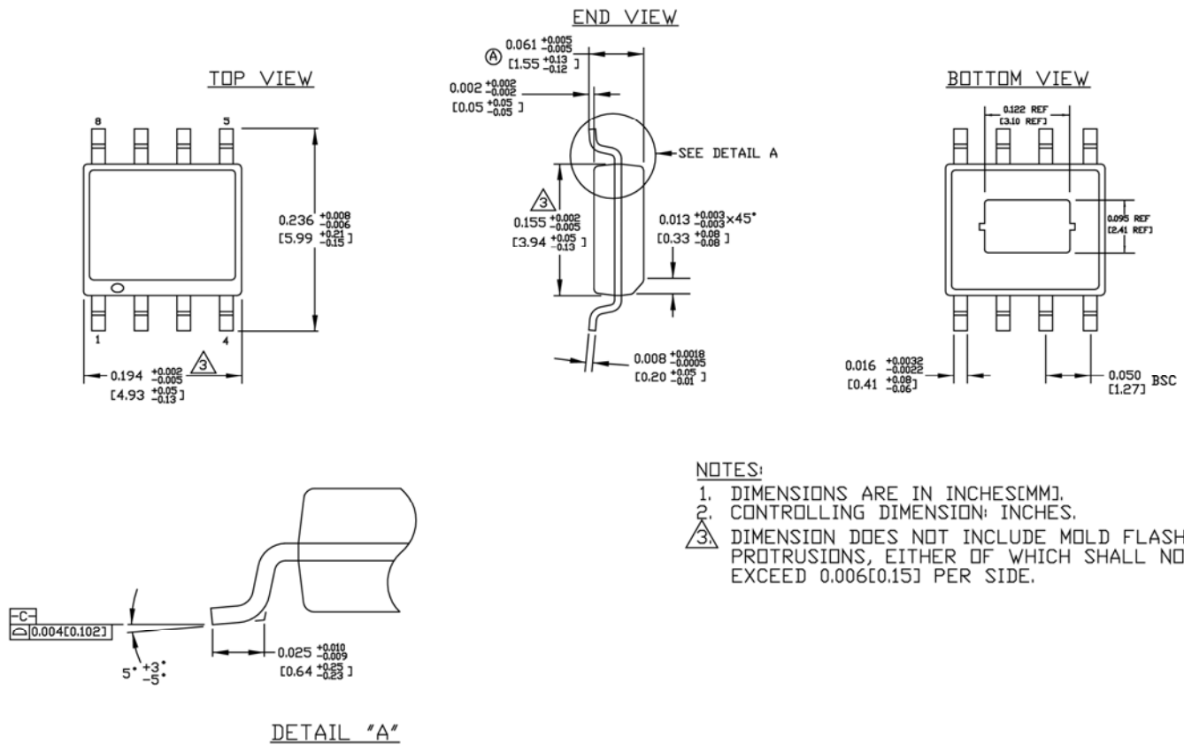
8-Pin ePad SOIC (ME)
