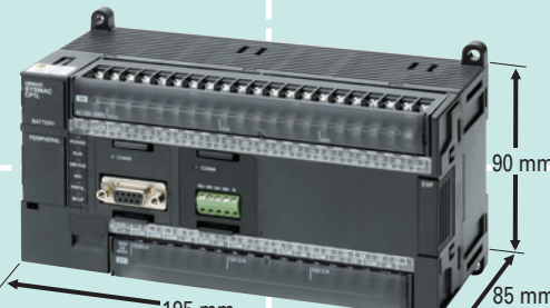
CP1L-M60D□-□
