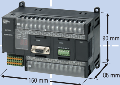
CP1H-40D
