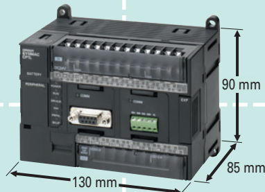
CP1L-M30D
