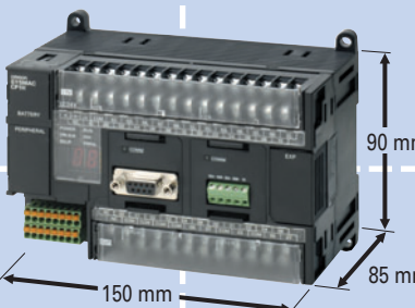
CP1H-40D
