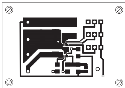
TOP LAYER
